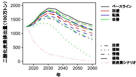
図 1-14 2015 年から 2060 年の中国の運輸部門からの CO 2 排出経路
