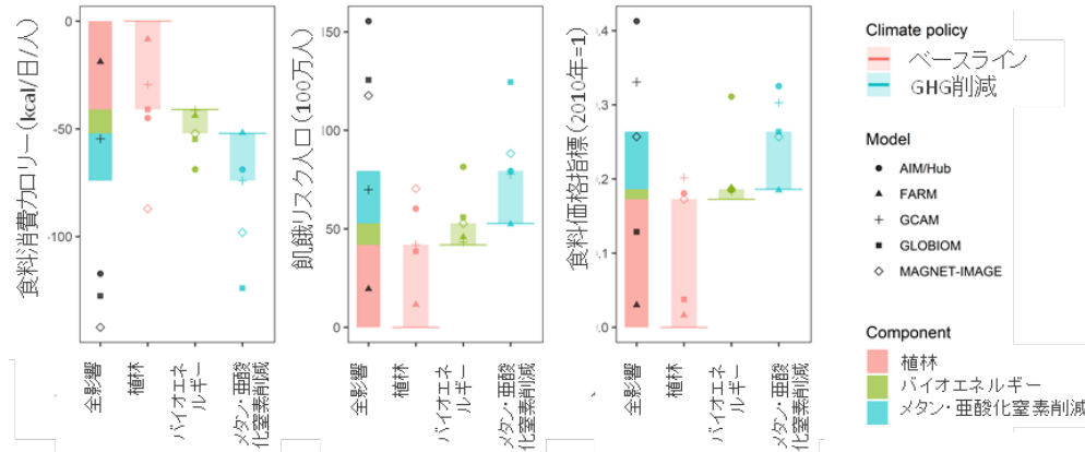
図 1-13 世界全体の 2050 年脱炭素シナリオの飢餓リスクの要因分解
